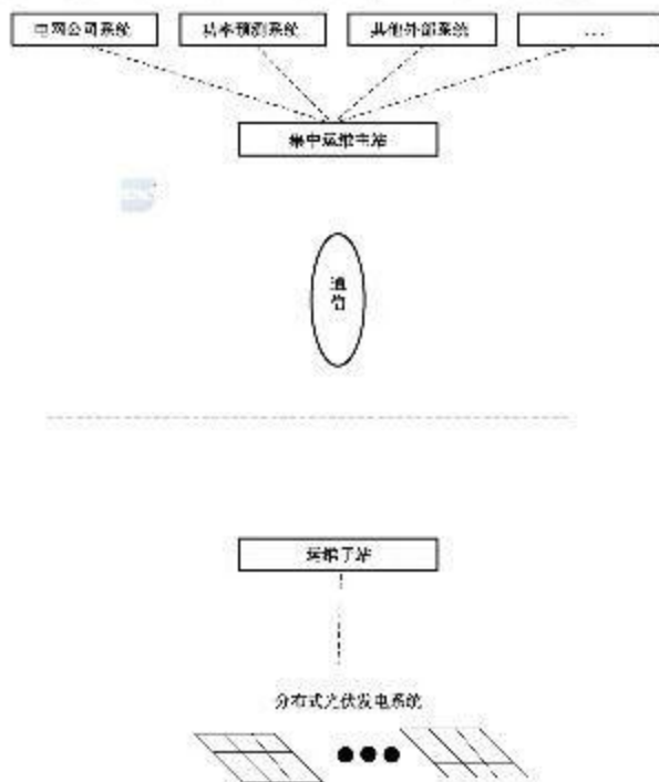
图 C.1 集中运维系统结构图
